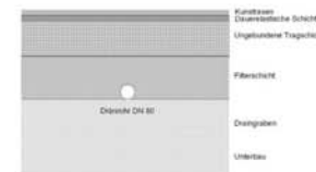
Aufbau Kunstrasen M 1 : 10
